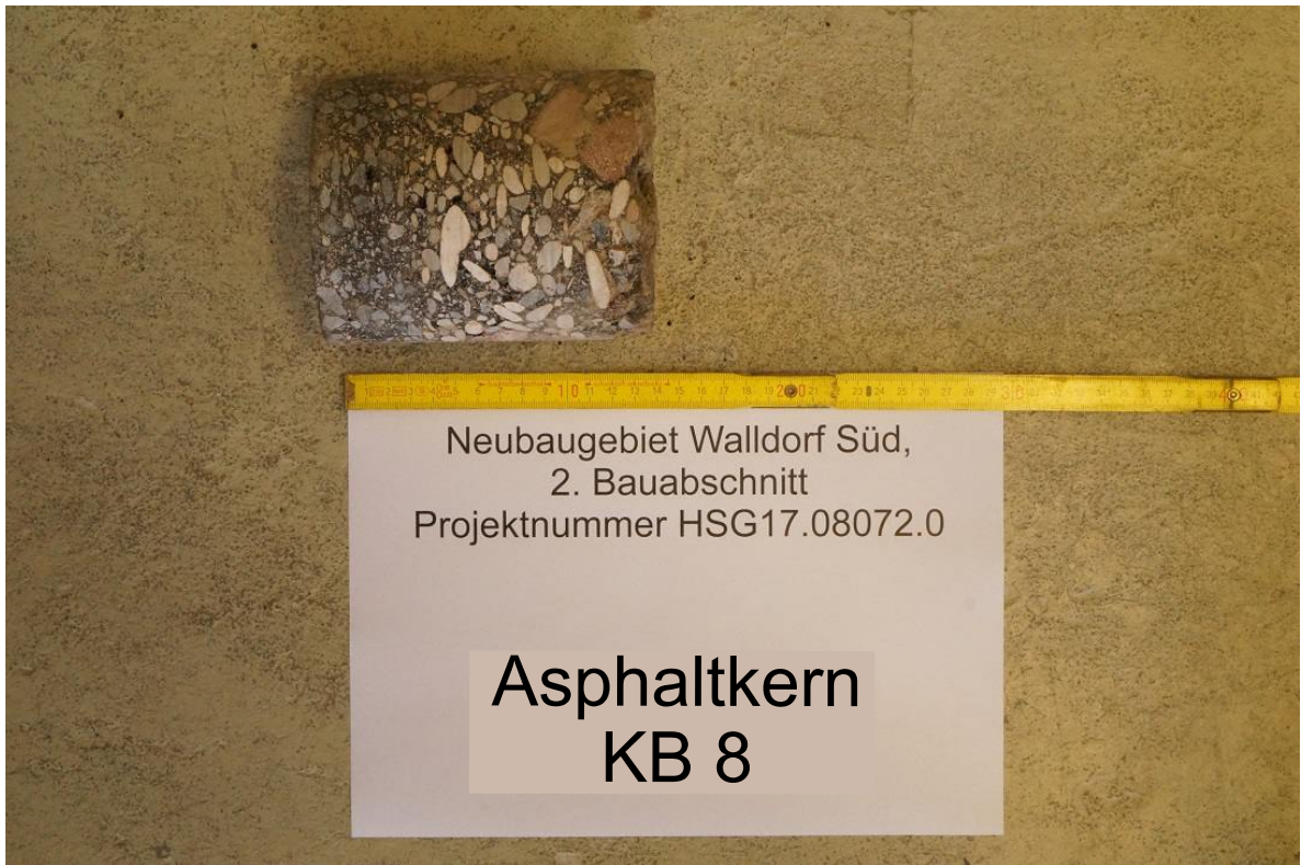
Bild 17: Asphaltkern KB 8
