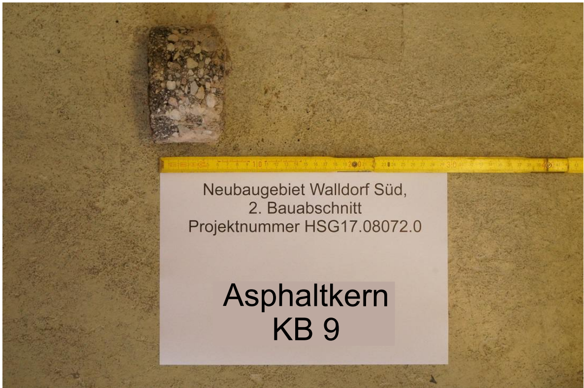
Bild 19: Asphaltkern KB 9
