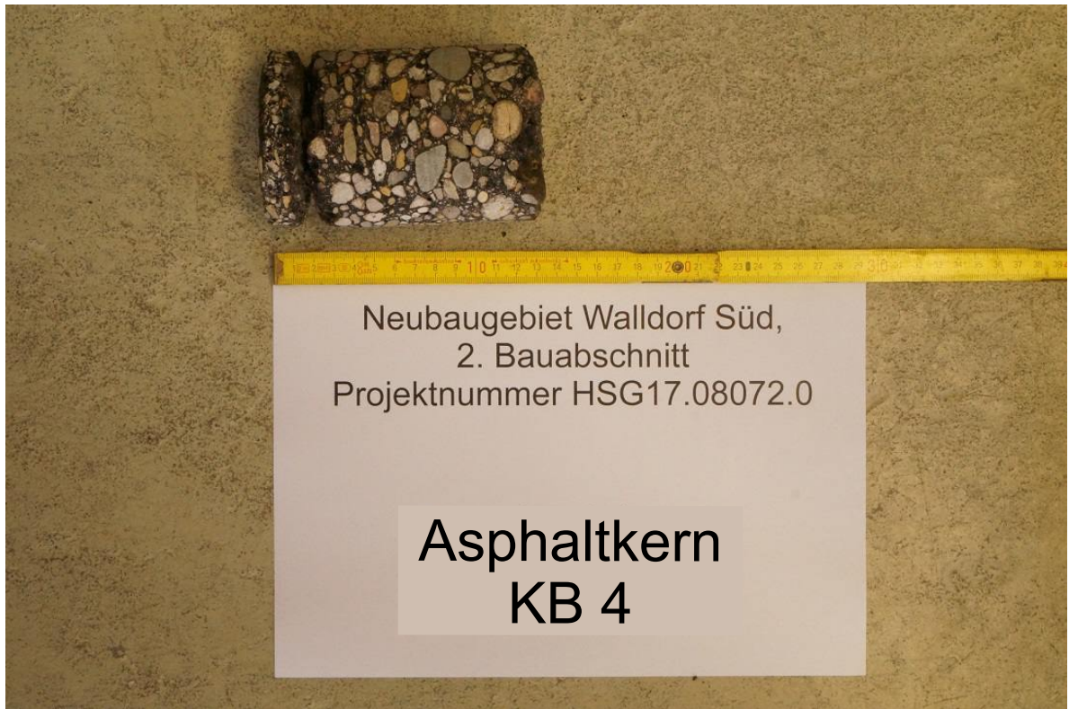
Bild 9: Asphaltkern KB 4
