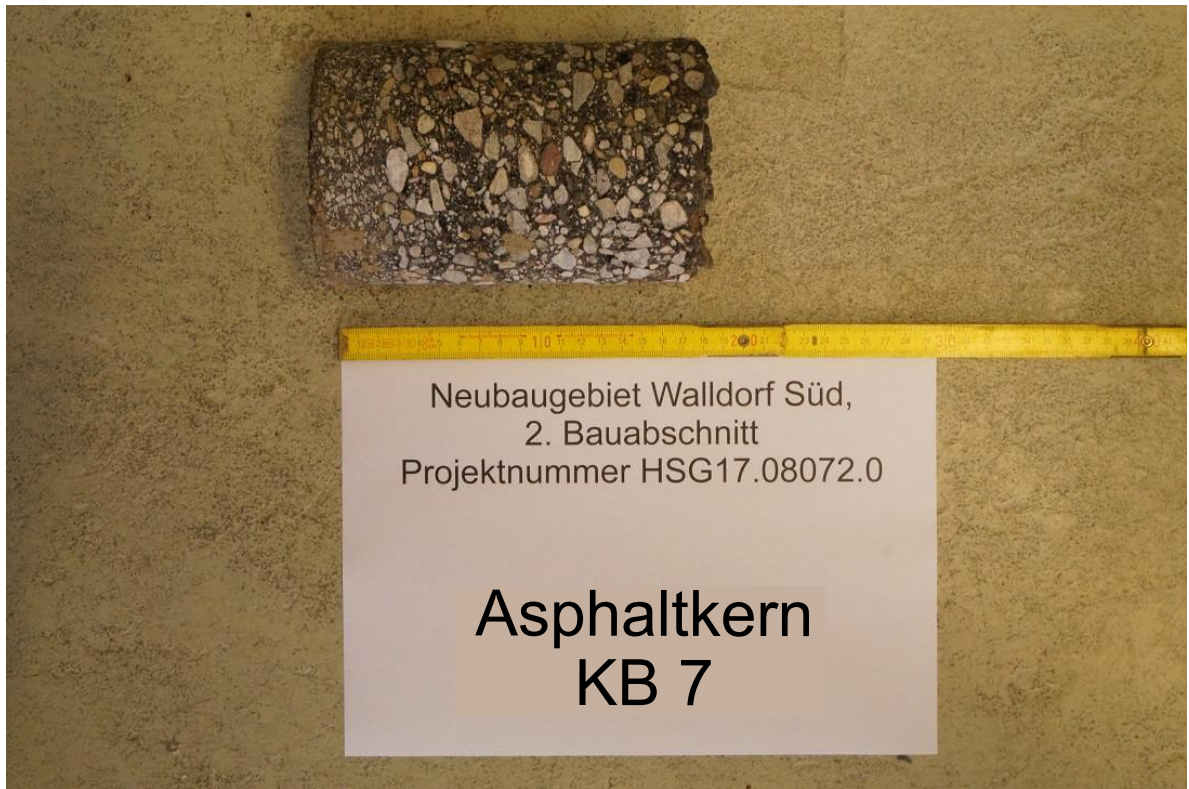
Bild 15: Asphaltkern KB 7
